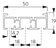
SG 10123 Profil 3-läufig
