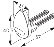
SG 4944 Enddeckel
