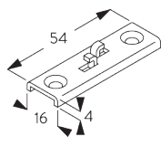
SG 6124 КРОНШТЕЙН
