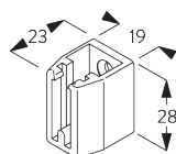
SG 3602 настенная опора
