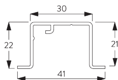
SG 11230 пазовый профиль
