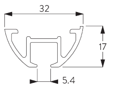
SG 6170p профиль
