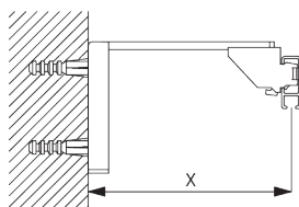
Smart Fix SG 11200 - SG 11205 и кронштейн SG 3603: необходимо использовать крепеж SG 10492 (M4x8).
