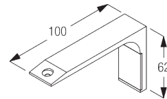
SG 11669 дизайн-кронштейн
