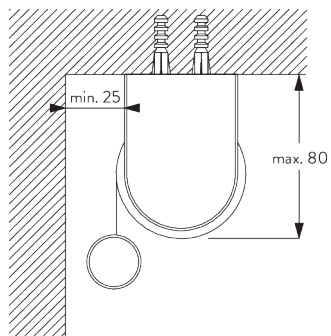
Кронштейны
