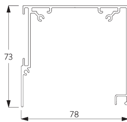
SG 11433 Корпус 73 мм
