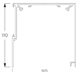
SG 11533 Корпус 110 мм
