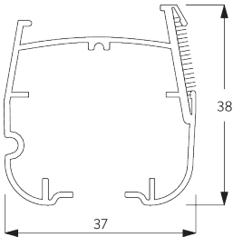
SG 2301 Velcro профиль
