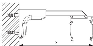
Universal Smart Fix SG 11154 - SG 11156 и кронштейн SG 2521: крепеж SG 10492 (M4x8).
