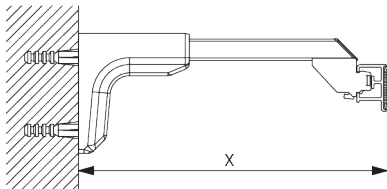
Universal Smart Fix 11154-11156 и кронштейн SG 3603: крепеж SG 10277 (M4x12).
