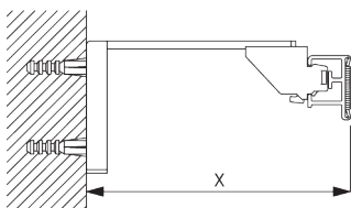
Smart Fix SG 11200 - SG 11205 и кронштейн SG 3603: крепеж SG 10492 (M4x8).
