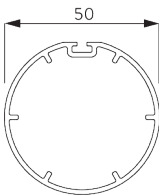
SG 2352 профиль ø 50 mm
