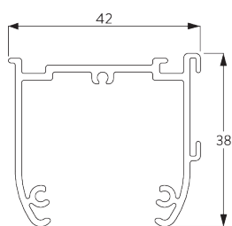
SG 2321 профиль
