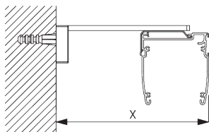
Square Smart Fix SG 11210 - SG 11214 и кронштейн SG 2521: крепеж SG 10395 (M4x6).
