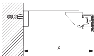
Square Smart Fix SG 11210 - SG 11215 и кронштейн SG 3603: крепеж SG 10492 (M4x8).
