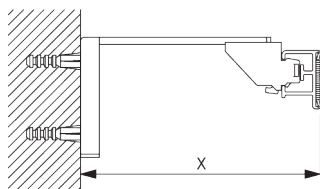
Smart Fix SG 11200 - SG 11205 и кронштейн SG 3603: крепеж SG 10492 (M4x8).
