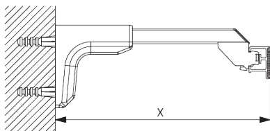
Universal Smart Fix SG 11154 - SG 11156 и кронштейн SG 3603: крепеж SG 10277 (M4x12).
