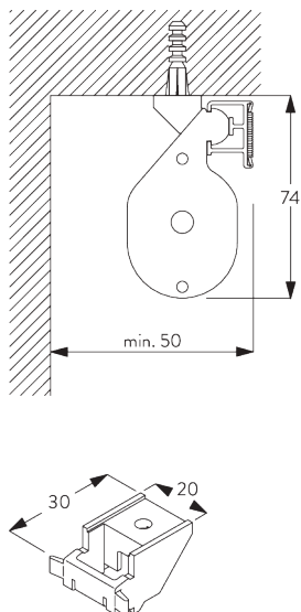
SG 3603 кронштейн
