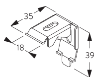
SG 2302 кронштейн
