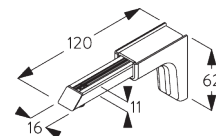
SG 11154 Universal Smart Fix 120 мм
